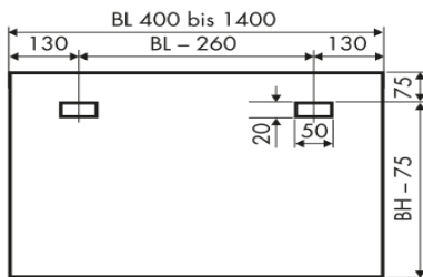
Haltetaschen Anordnung
